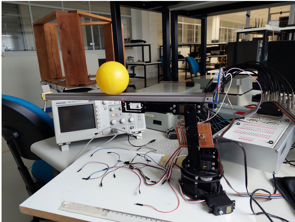
Abbildung 1: Versuchsaufbau Ball and Beam System
